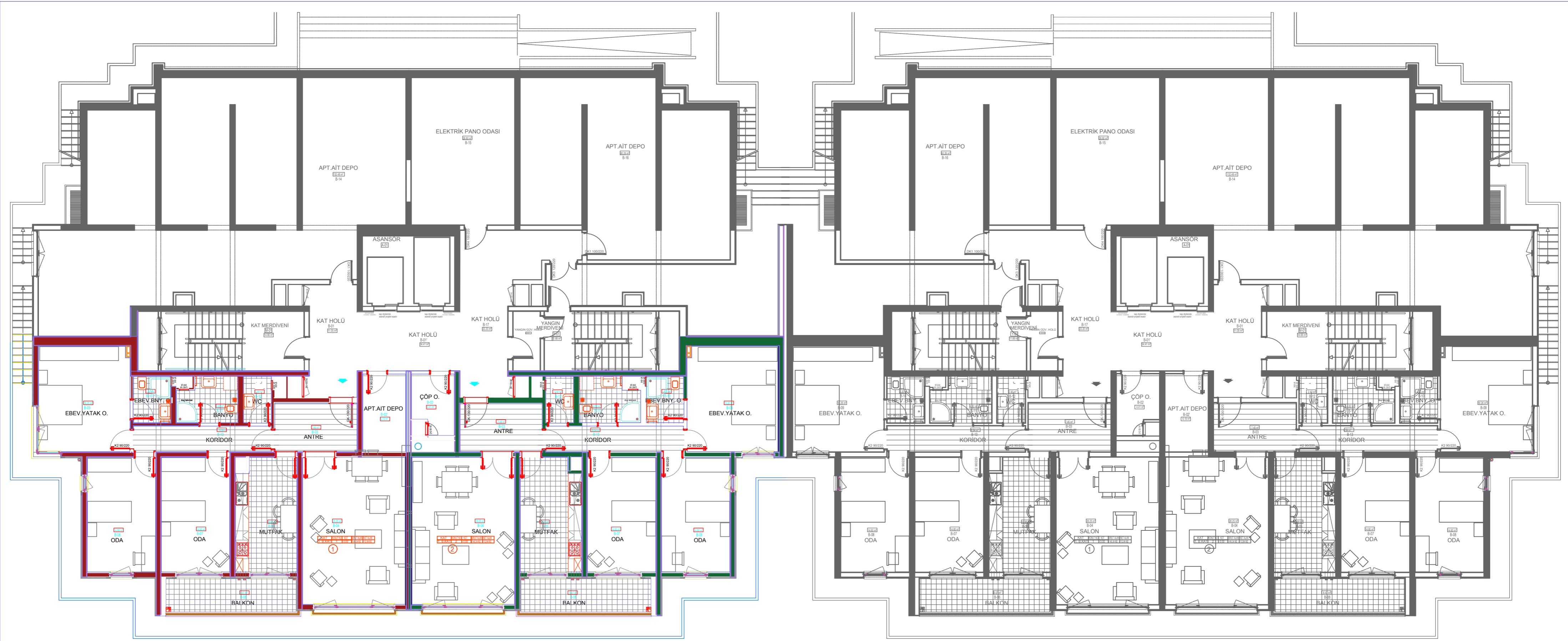
ANKARA SINCAN SARAYCIK MAHALLESİ G.Ö.B. KENTSEL DÖNÜŞÜM PROJESİ SC TİP BLOK BODRUM KAT PLANI
